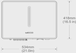
Serie 20 kW
